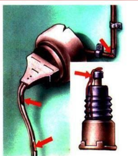
Неисправность электропроводки
